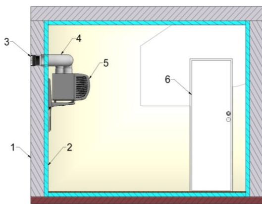
Schnitt
